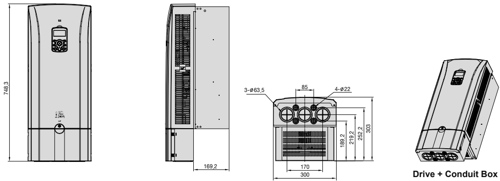
Drive + Conduit Box
