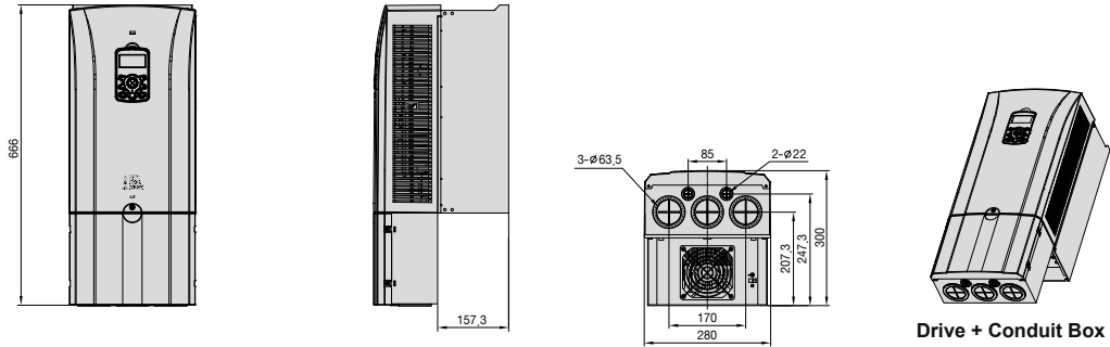
Drive + Conduit Box
