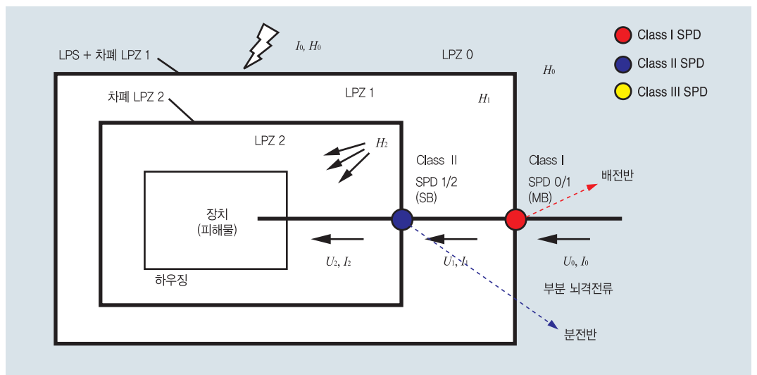
공간차폐물과 협조된 SPD 보호를 이용한 LEMS - 전도성 서지와 방사자계에 대해 잘 보호된 장치 장치-
