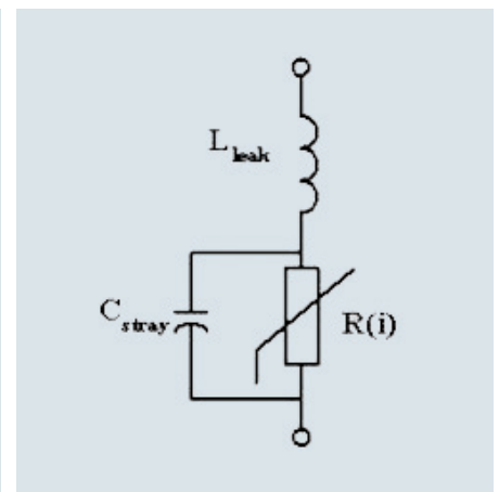
MOV 등가회로
