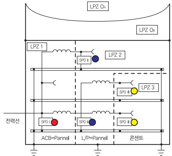
전원시스템의 SPD 적용 예
