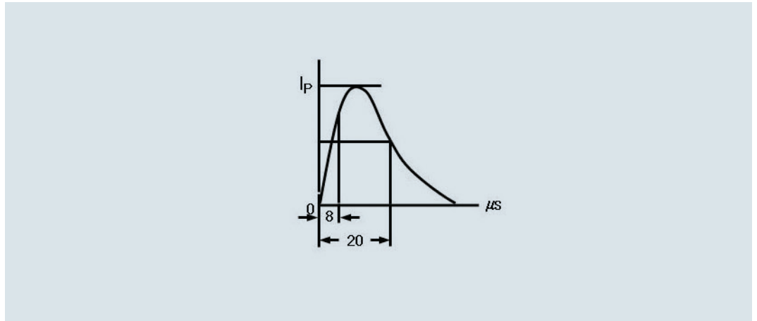
서지전류 파형 파형
