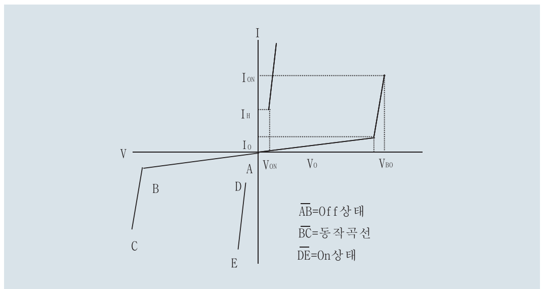
실리콘억제소자의 V-특성
