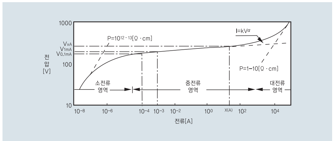
산화아연 바리스터(MOV)의 V-I 특성
