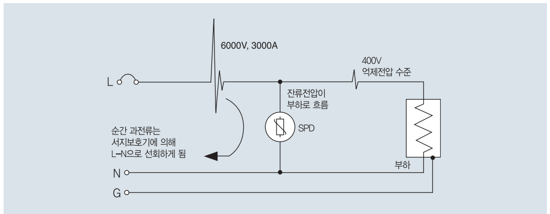
SPD의 서지억제 개념도
