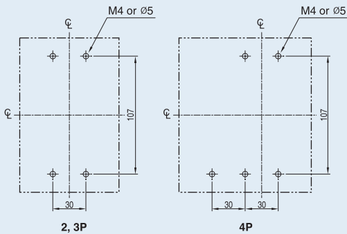
패널설치치수
