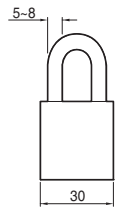
자물쇠의 크기
