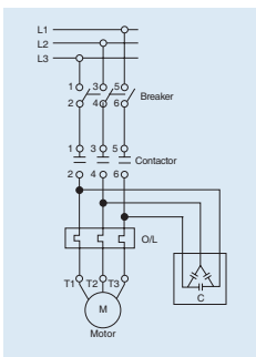
콘덴서 회로
