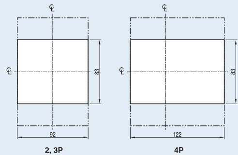
패널커버절단치수
