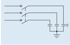
콘덴서 회로
