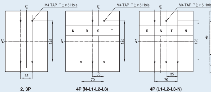
패널설치치수
