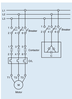
정상적인 회로
