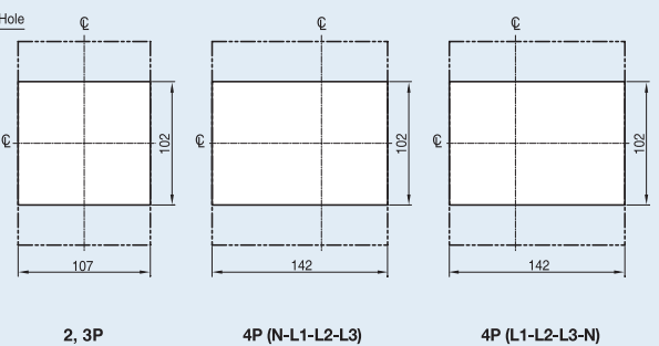
패널커버절단치수
