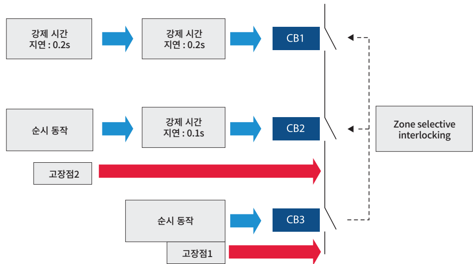
그림 2. ZSI의 원리
