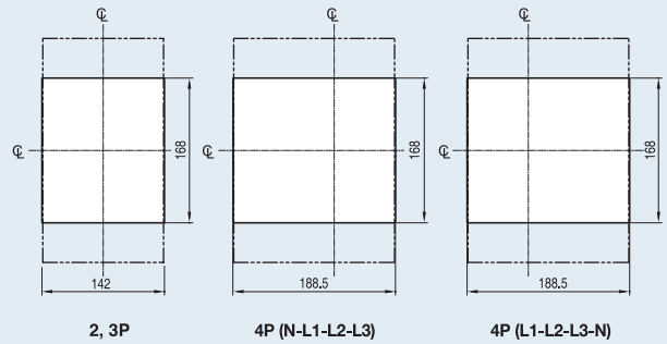
패널커버절단치수
