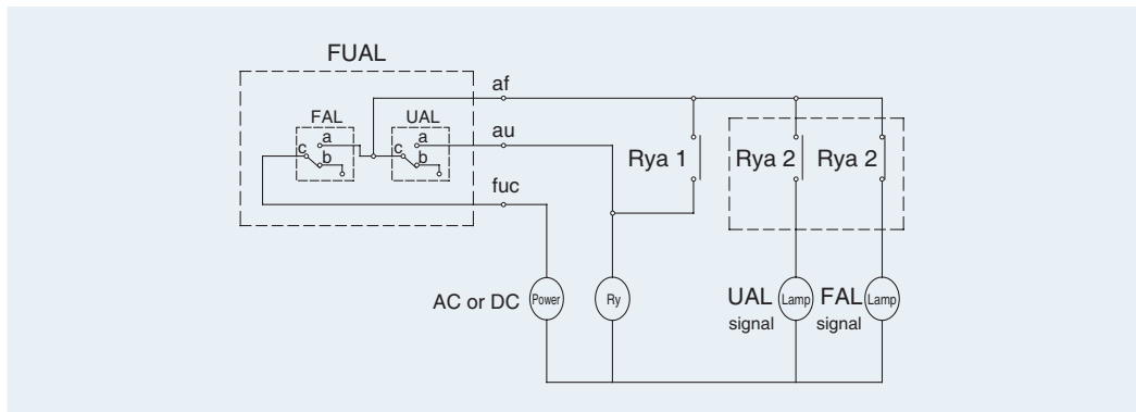
그림 : FUAL용 자기유지회로의 예
