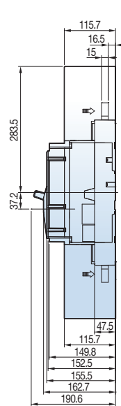
<TS1000NA 3P>
