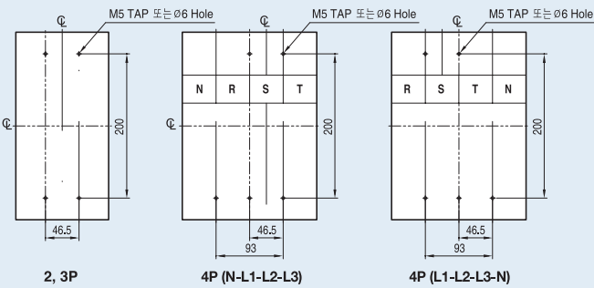
패널설치치수
