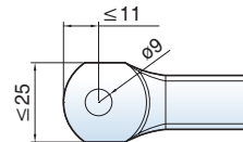
단자 치수
