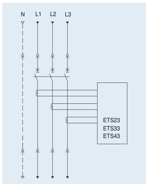
트립장치 ETS23, ETS33, ETS43이 장착된 3극형 MCCB의 경우
