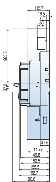
<TS1000NA 4P>
