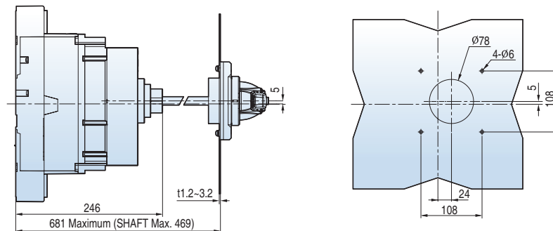
도어커팅치수
