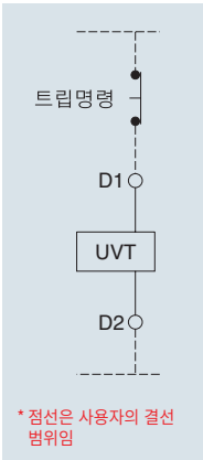
결선도
