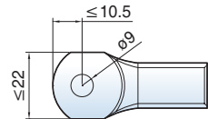
단자 치수
