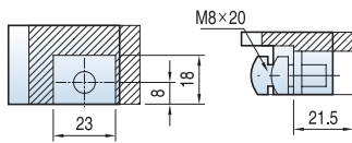
단자부상세도
