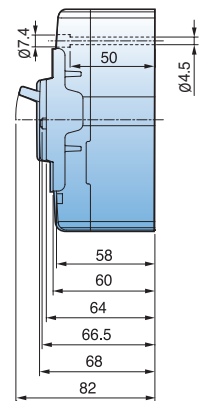
(외형도 1)
