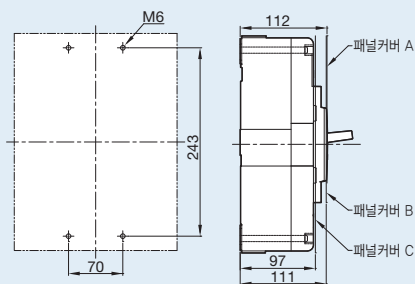
패널설치치수
