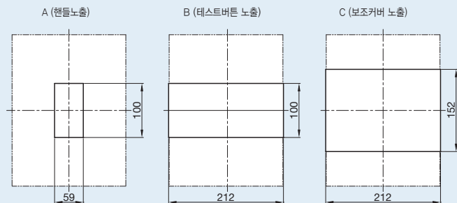
패널커버절단치수
