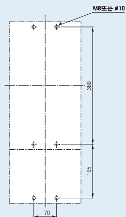
패널설치치수
