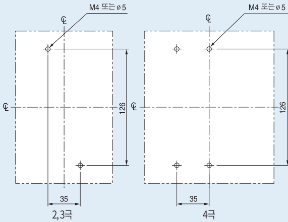
패널설치치수
