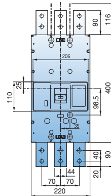
(외형도 6)
