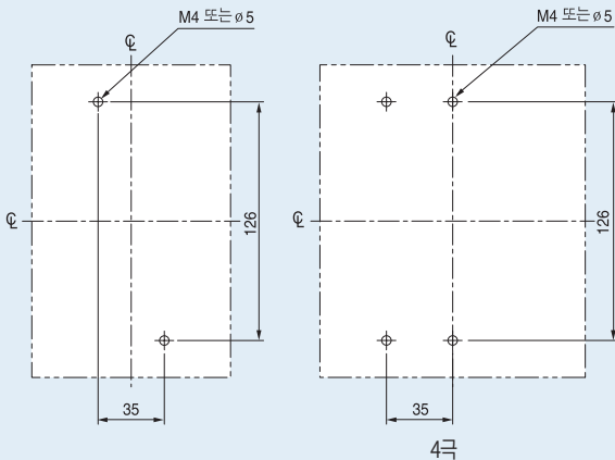
패널설치치수
