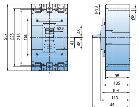
(외형도 4)
