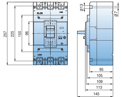
(외형도 4)
