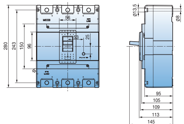
(외형도 5)
