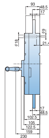
(외형도 6)
