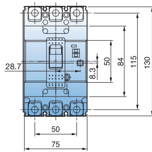
(외형도 1)
