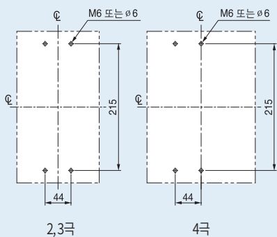
패널설치치수
