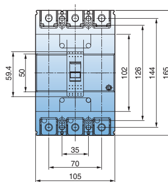
(외형도 3)
