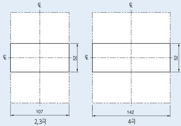
패널커버절단치수
