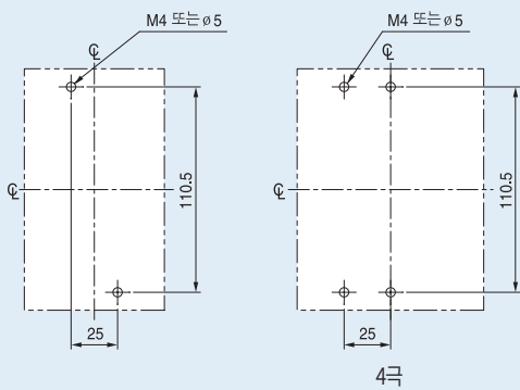
패널설치치수
